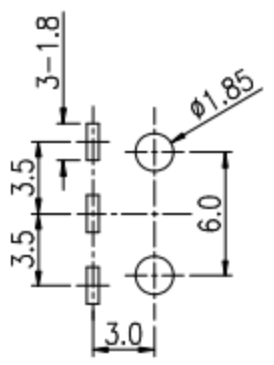
P.C.B LAYOUT
